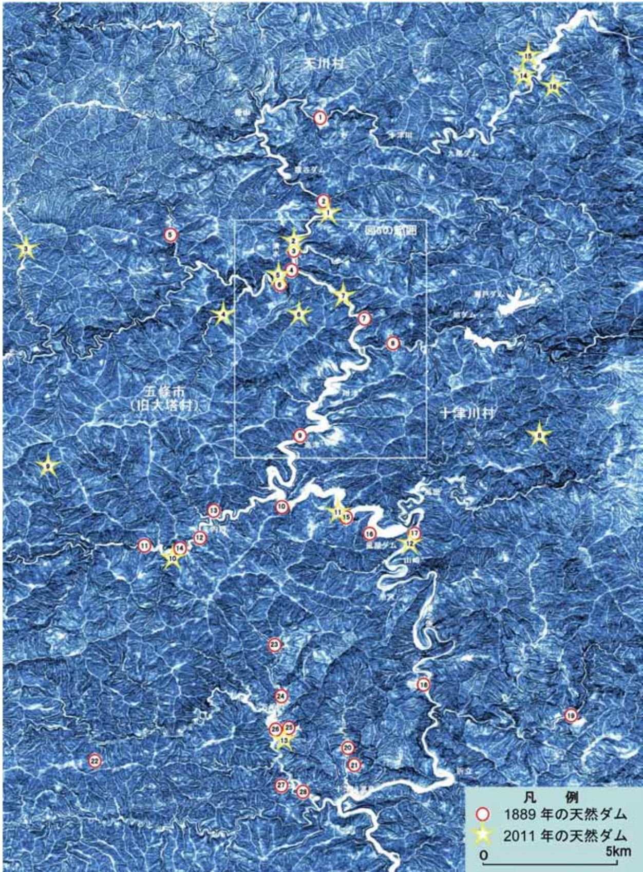
図2 紀伊半島中央部・十津川流域の1889年と2011年災害における天然ダム形成位置。 Fig.2 Distribution of landslide dams in 1889 and 2011 disaster on the Totsu River, central Kii Peninsula
