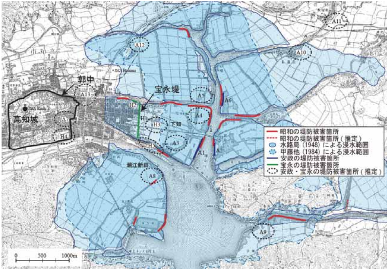
図 8 安政や宝永南海地震による堤防被害と昭和南海地震による堤防被害の位置の比較.
