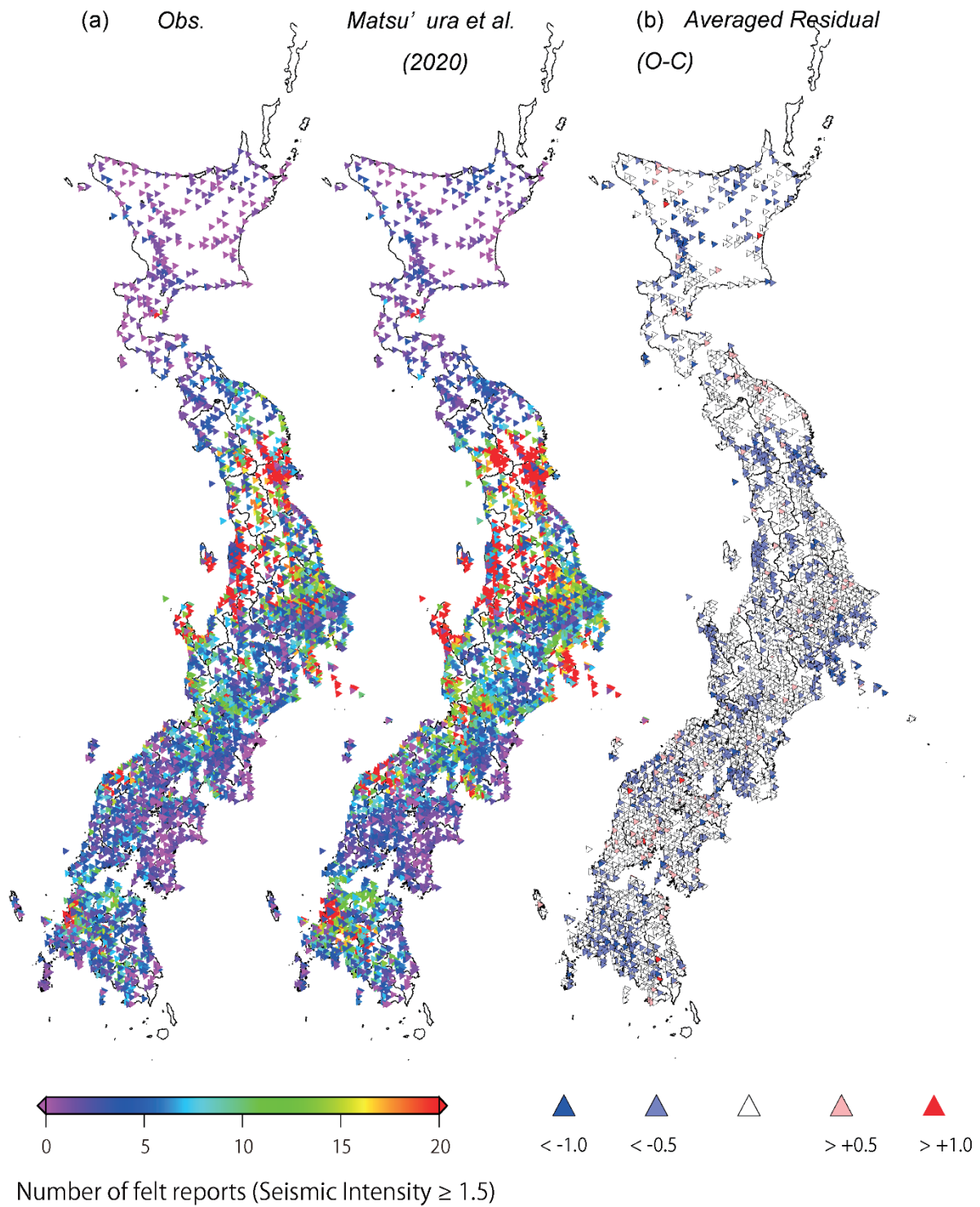
図 5. (a) (左)2000 年～2010 年に発生した最大震度 3 以上を観測した浅発地震(図 1)による, それぞれの観測点における有感地震数の分布と, (右)距離減衰式によって計算された有感地震数の分布の比較. (b) それぞれの観測点における震度残差(観測値-計算値)の平均値.
