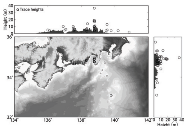
図 1. 明応東海地震の計算津波高と津波痕跡高。丸は実測された津波痕跡高、灰色の棒が最寄りの海岸線における計算浸水高をそれぞれ示す。
