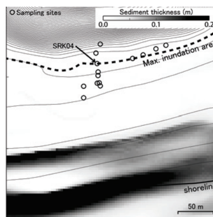
図 2. 静岡県湖西市白須賀における最大浸水範囲と津波土砂移動数値解析による土砂堆積量。地形コンターは 1m 間隔である。
